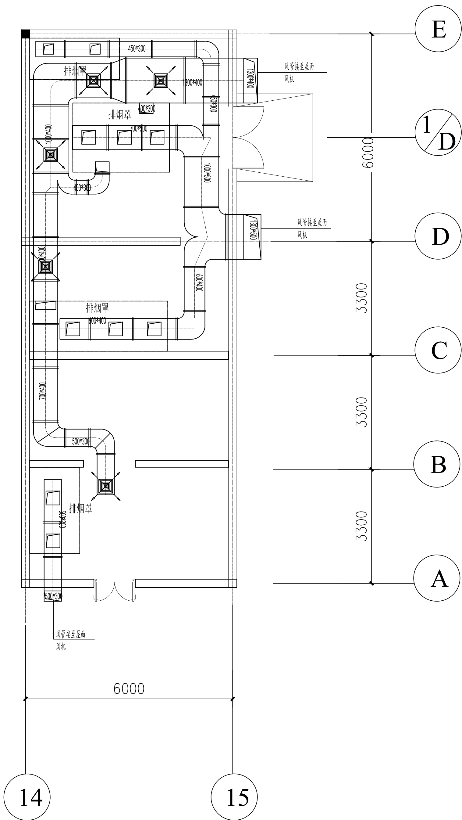
上海海事大学港湾校区实训项目通排风系统
